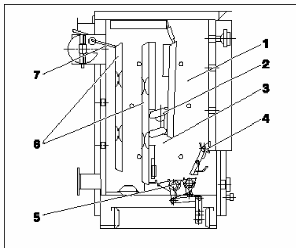
Рис. 2 Котел в разрезе, здесь тип 24
